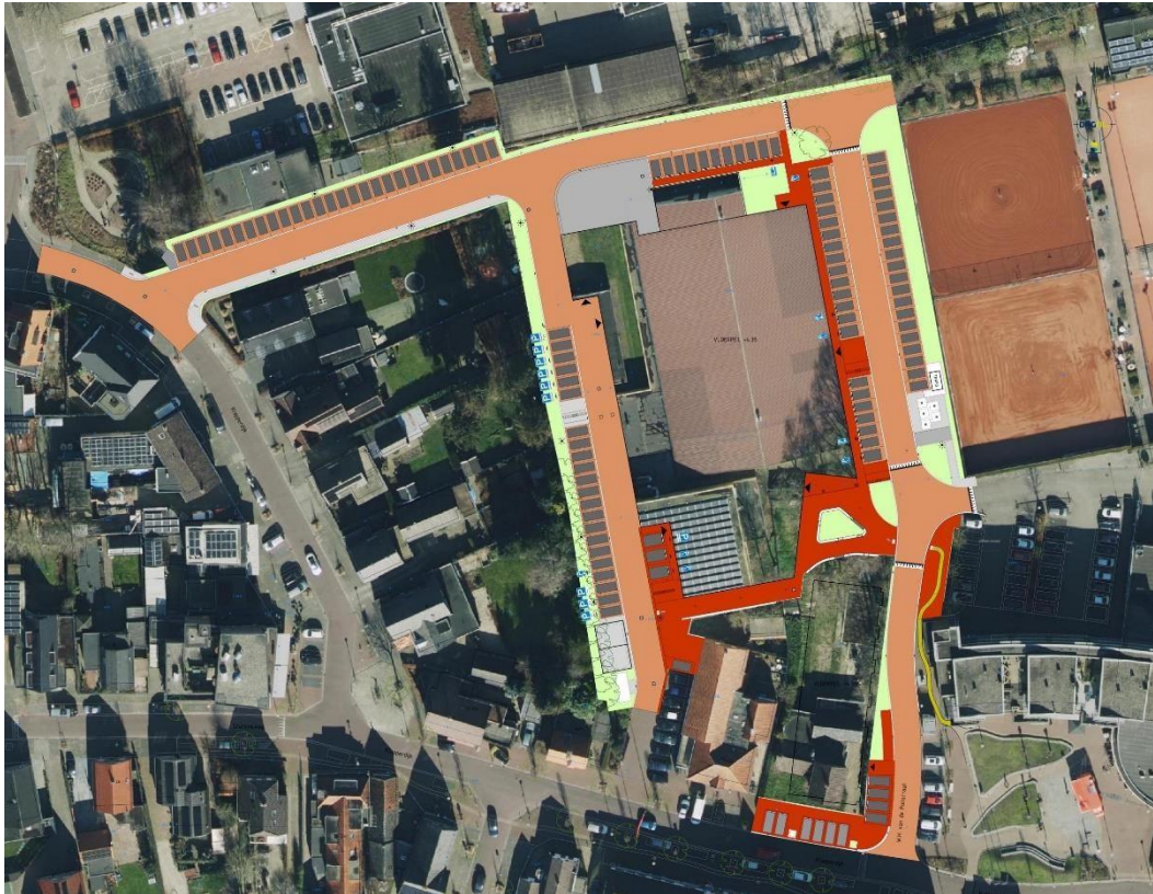
Afbeelding 2; Plattegrond civiele ruimte rondom MFA Wapenveld.
